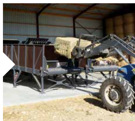
Mélangeuse à vis verticale
